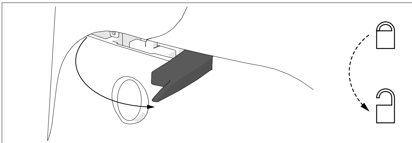
Fig. 5 IT - Sbocco del motoriduttore EN - Gearmotor release FR - Déblocage du motoréducteur ES - Desbloqueo del motorreductor
