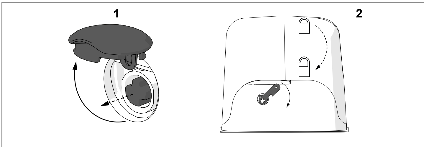
Fig. 4 IT - Sbocco del motoriduttore EN - Gearmotor release FR - Déblocage du motoréducteur ES - Desbloqueo del motorreductor
